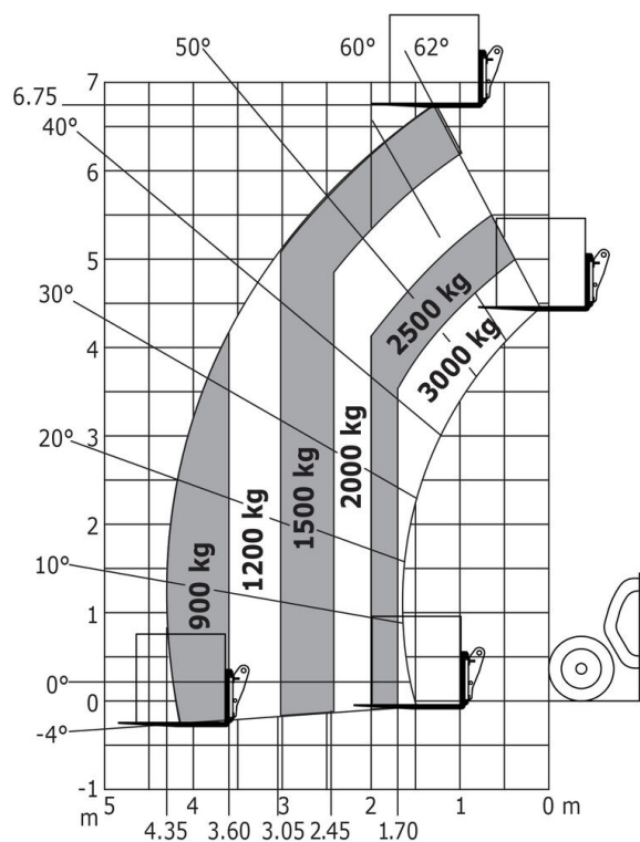
Rough terrain load chart (EN 1459 B) Metric
